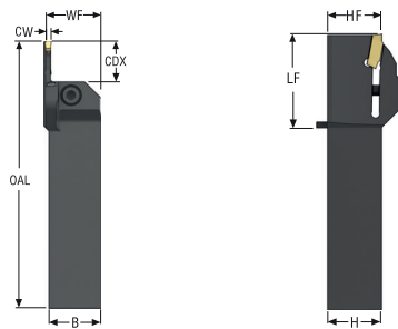
CFOR...L...JETI, CFOL...R...JETI
