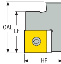
CT-PLANR/L
