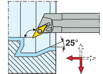
PVPNR/L KAPR = 117,5 °
