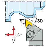
CDNNN KAPR = 62,5 °
