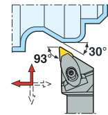
DDJNR/L...JETI KAPRI = 93,0°
