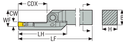
CFOR...L...JET, CFOL...R...JET
